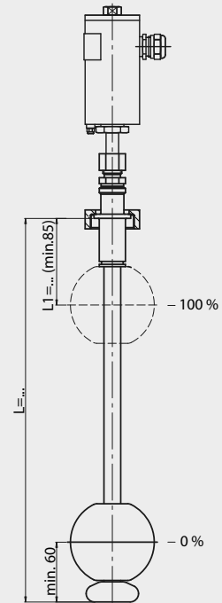
Ingold connection with box Type AVVE ...
